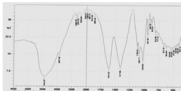
Gambar 3. Hasil analisis FTIR alginat dari alga coklat jenis Sargassum sp (Anshar & Wahid, 2013)
