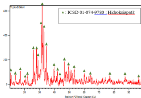
Gambar 1. Hasil analisis XRD sintesis HAp dari tulang ikan dengan metode sol-gel (Anggresani, et al., 2019)
