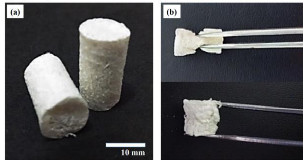
Gambar 4. (a) bentuk 3D perancah berpori berbasis HA/alginat dan (b) sifat elastis perancah berpori (Afriani, 2015)
