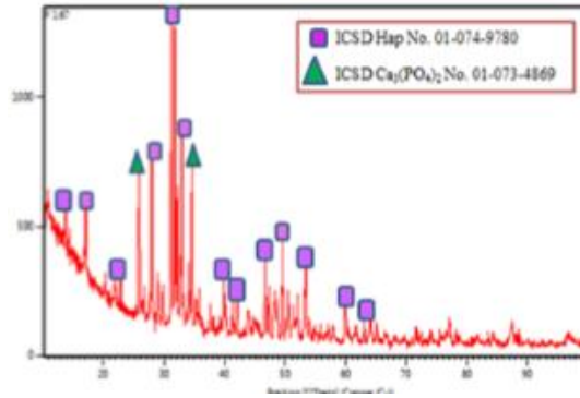
Gambar 2. Hasil analisis XRD sintesis HAp dengan metode presipitasi (Anggresani, et al., 2020)
