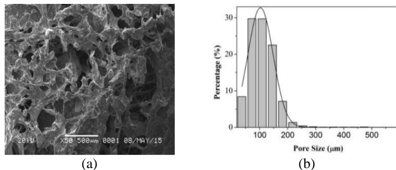
Gambar 5. Morfologi SEM perancah komposit HA/alginat (Afriani, 2015)
